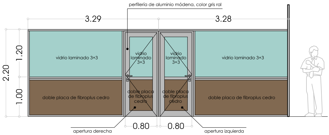
DETALLE T1 (ESC. 1:50)
