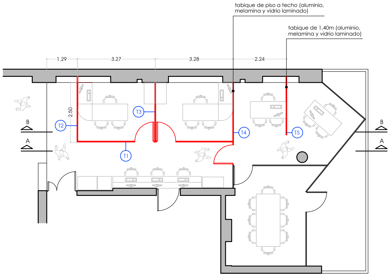
PLANTA OFICINAS (ESC. 1:100)
