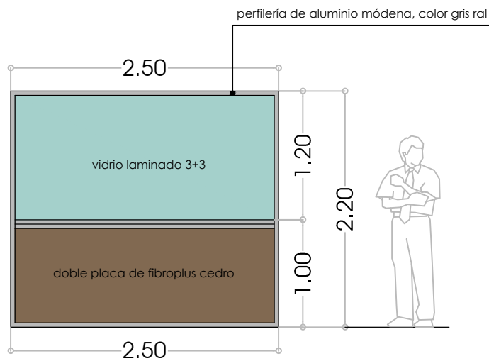
DETALLE T3 (ESC. 1:50)
