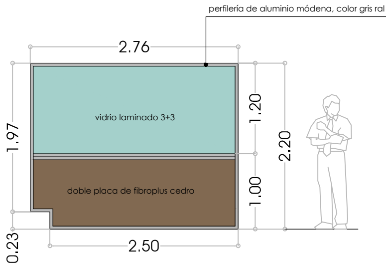
DETALLE T2 (ESC. 1:50)
