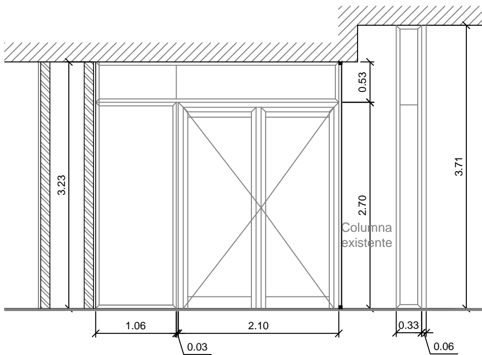
Vista esc. 1:50
